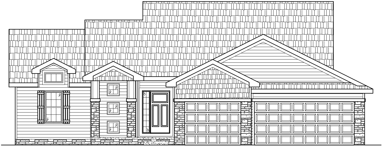
ELEVATION
